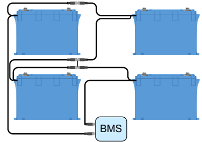
BMS-Anschluss für mehrere Batterien
